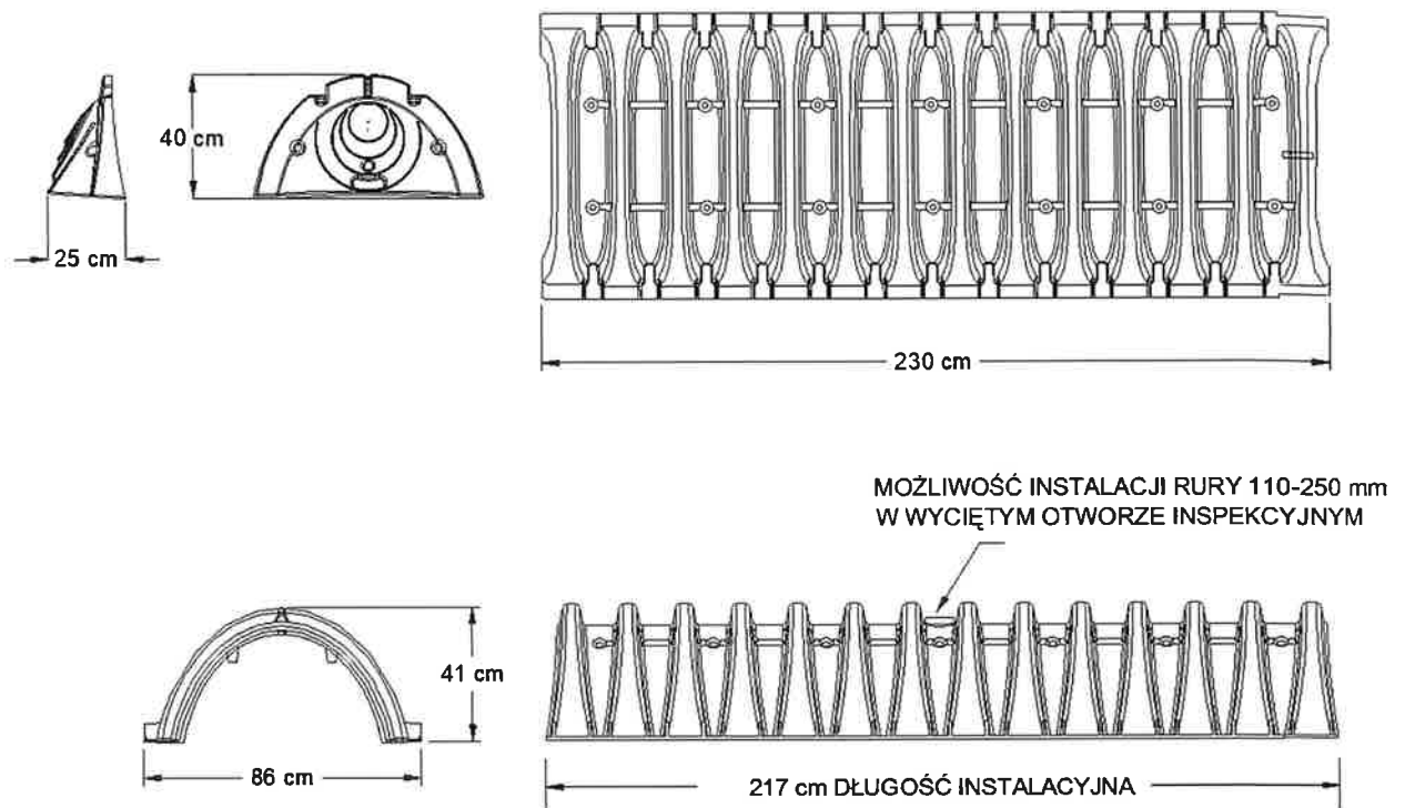
Rysunek Z-1 Komora drenażowa SC-310
