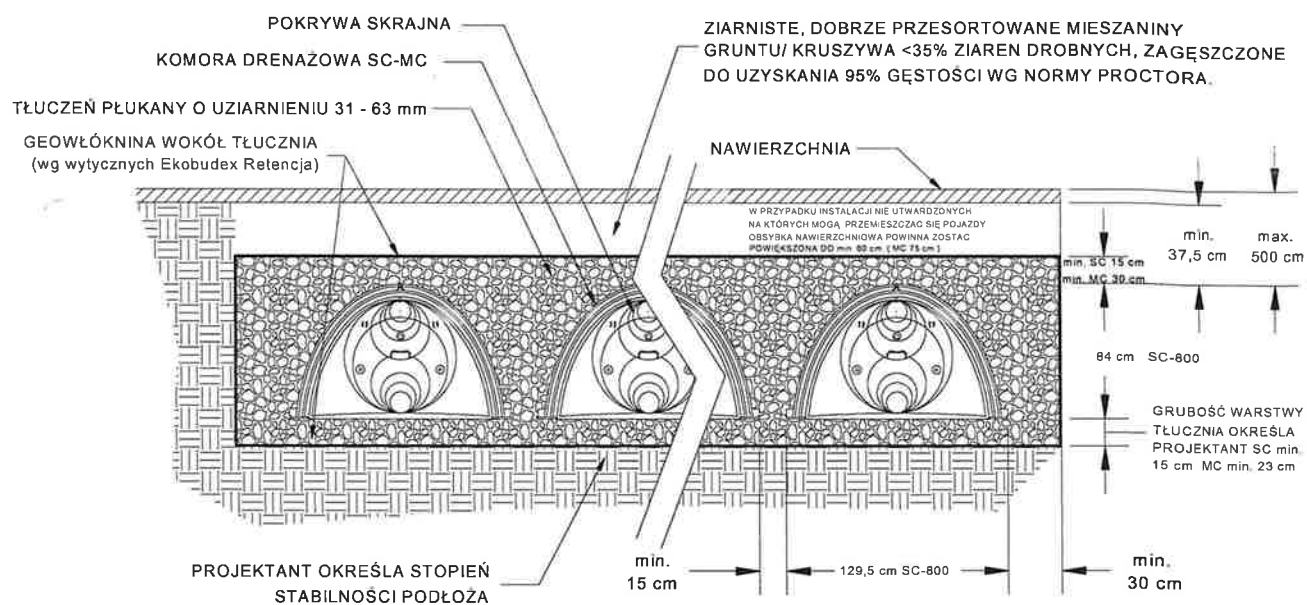
Rysunek Z-6 Przekrój poprzeczny komory drenażowej SC-800
