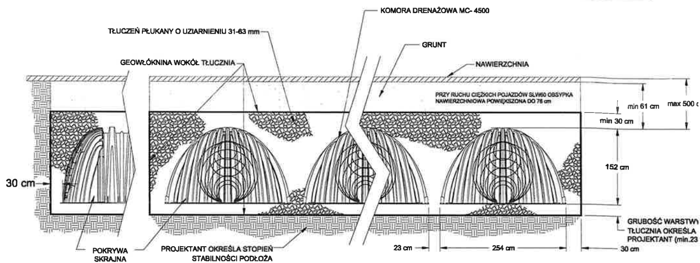
Rysunek Z-10 Przekrój poprzeczny komory drenazowej MC-4500
