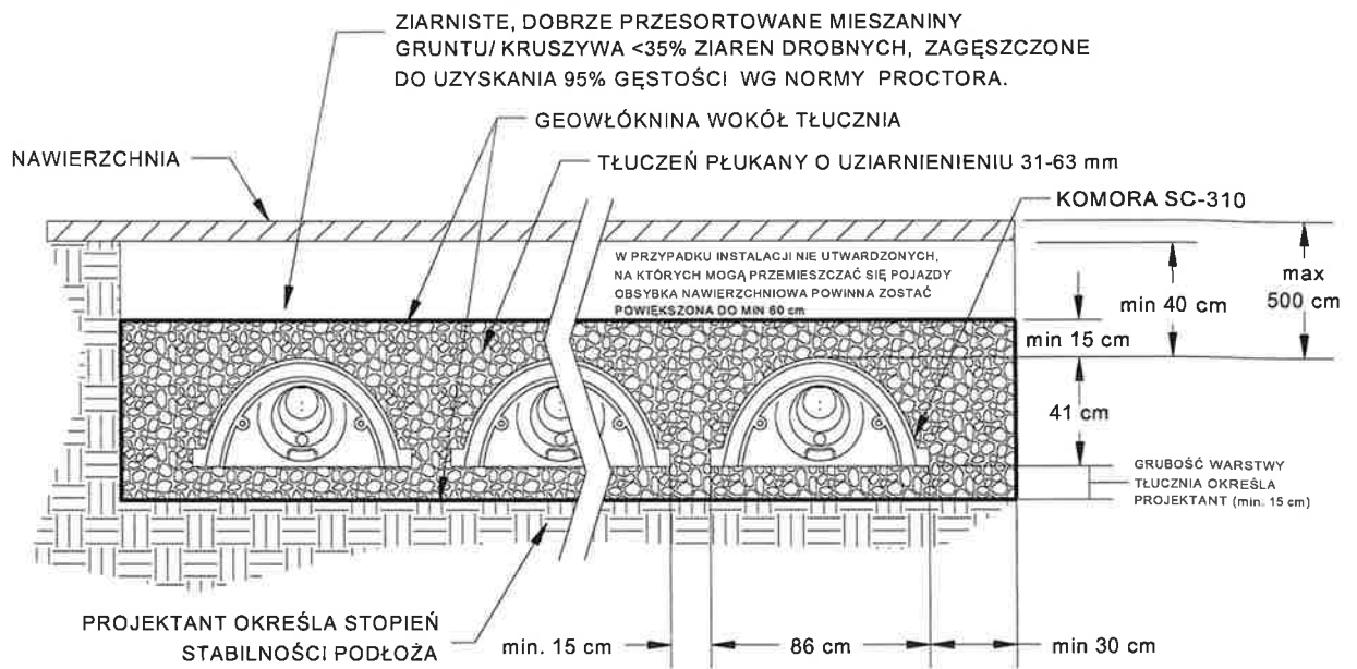
Rysunek Z-3 Przekrój poprzeczny komory drenażowej SC-310
