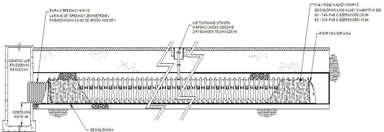
Rys. 1. Separator zanieczyszczeń Isolator™
