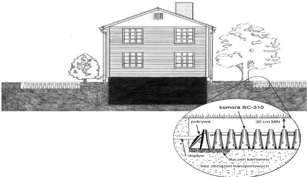
Rys. 10a. Wykorzystanie systemu dla domku jednorodzinnego
