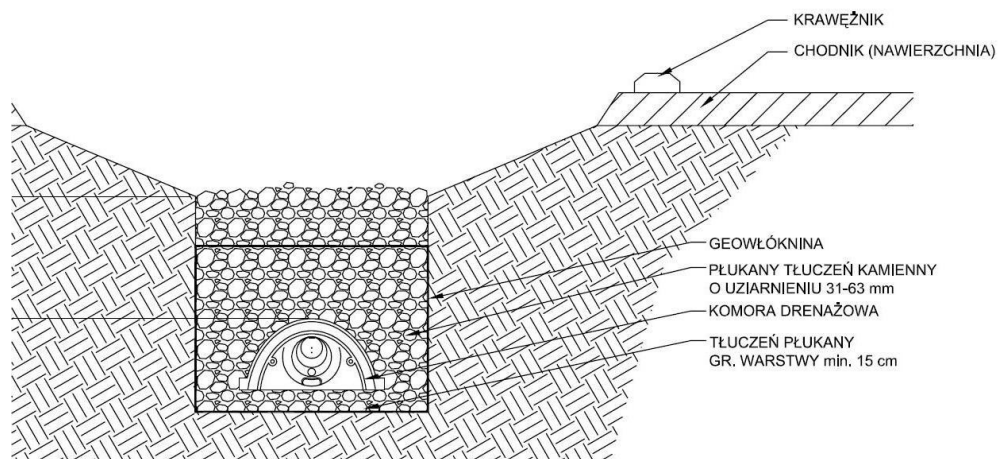
Rys. 15. Zastosowanie systemu komór drenażowych jako rów odwadniający
