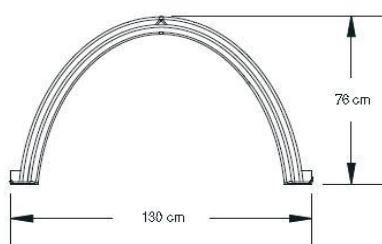
Rys. 4. Komora drenażowa SC-310 (bez zachowania skali)
