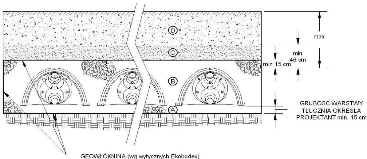
Rys. 11. Rozmieszczenie materiału wypełniającego
