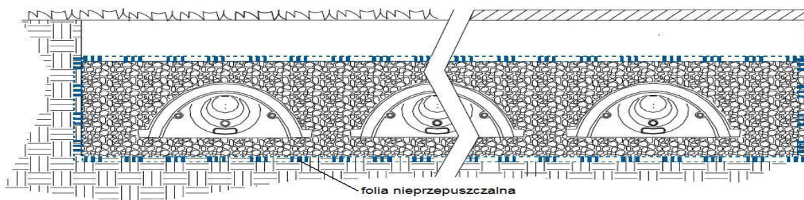
Rys. 9. Zbiornik szczelny utworzony z komór drenażowych SC za pomocą folii
