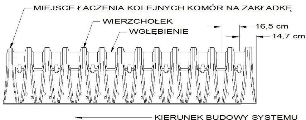
Rys. 5. Komora SC – Odległości pomiędzy połaďdowaniami
