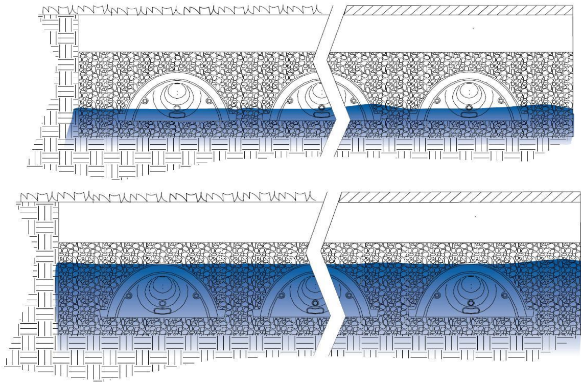
Rys. 9. Zbiornik szczelny utworzony z komór drenażowych SC za pomocą folii
