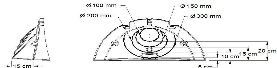
Rys. 6. Pokrywa skrajna komory typu SC-310
