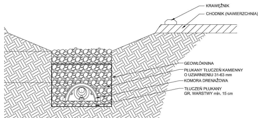
Rys. 10b. Zastosowanie systemu komór drenazowych SC jako rów odwadniający
