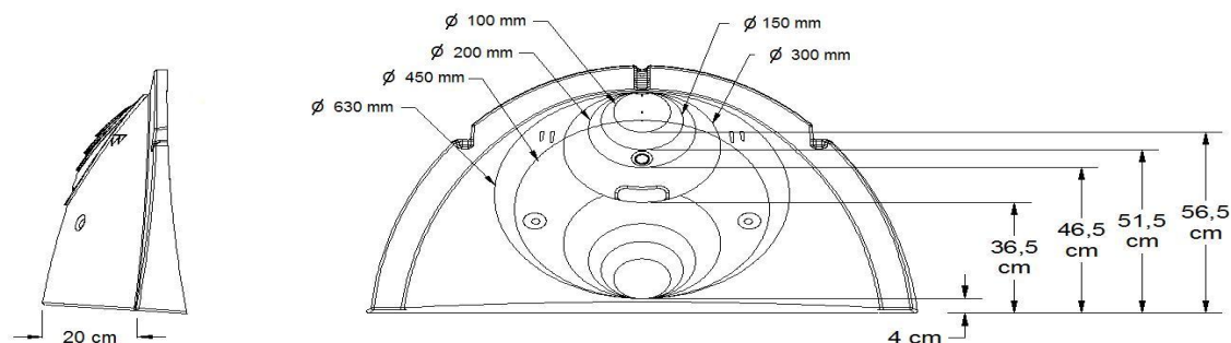
Rys. 7. Pokrywa skrajna komory typu SC-740
