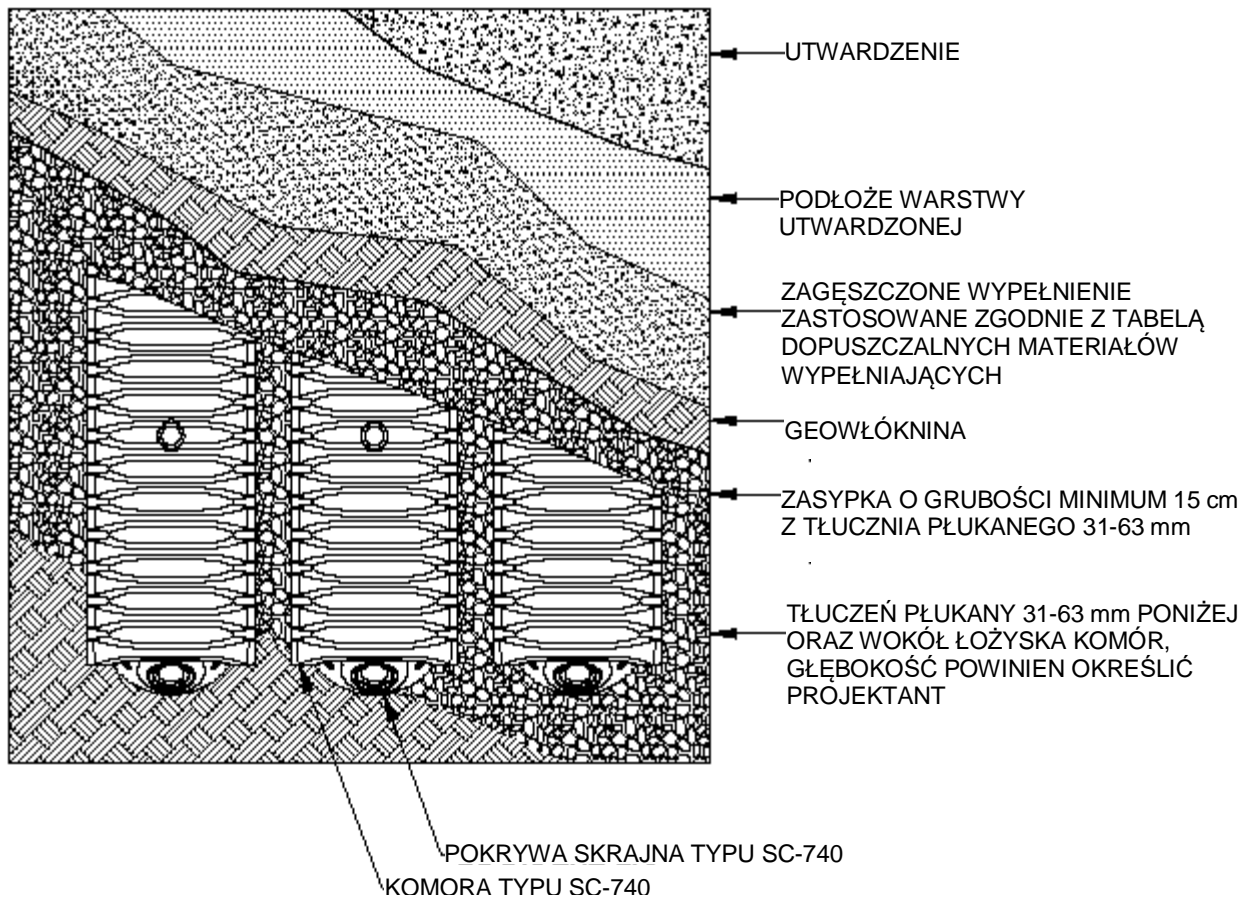
Rys. 13. Widok poziomy systemu komór
