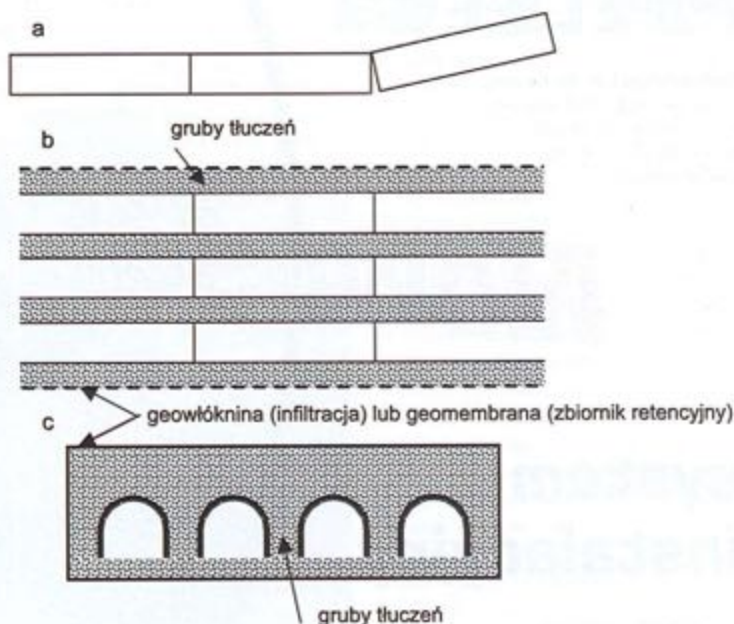
Rys. Charakterystyczny układ szeregowo-równoległy komór w obsypce z tłucznią: a) montaż komór, b) układ w rzucie, c) układ w przekroju.
