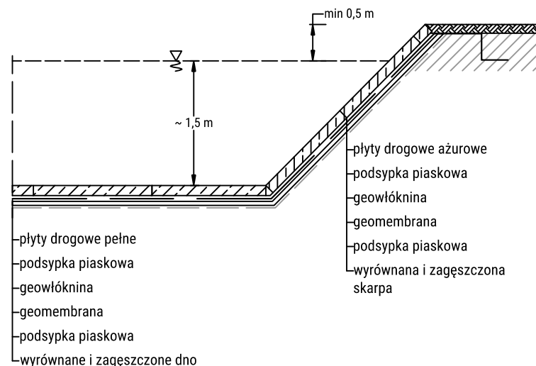
Przekrój przez zbiornik odparowujący
