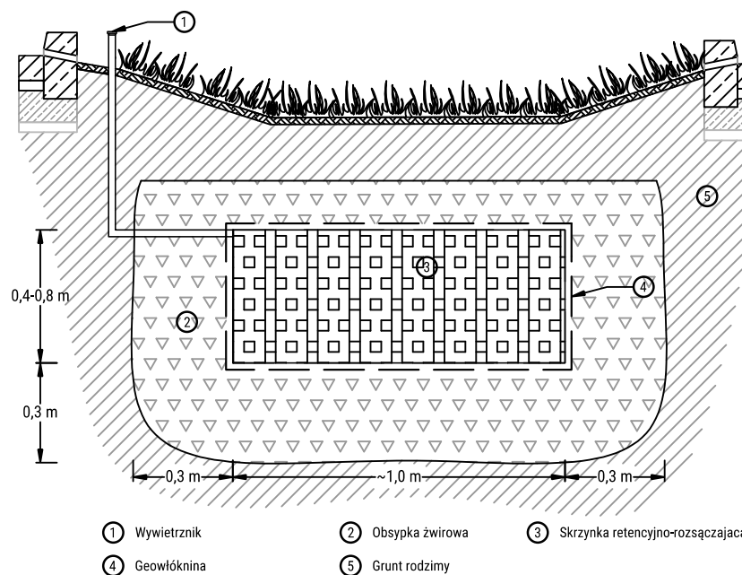
Przykład wykorzystania skrzynek retencyjno-rozsączających w muldziej chłonnej
