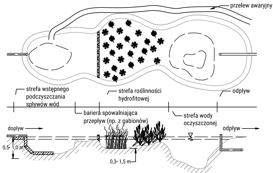
Obiekt hydrofitowy seminaturalny
