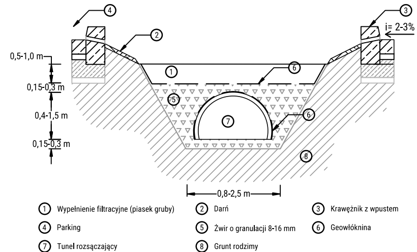
Przekrój przez rów odwadniający z zastosowaniem komór drenazowych
